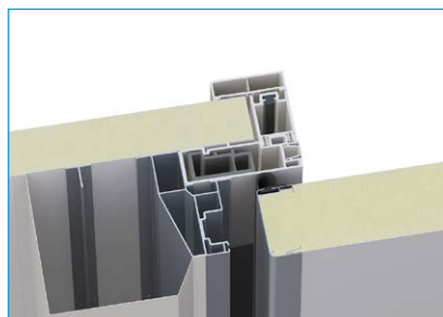
Section view of lower side blade Vista in sezione battente lato inferiore
